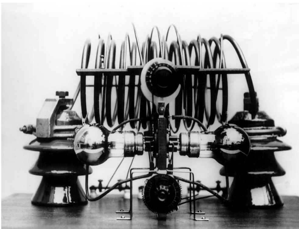
L'émetteur Mesny.
